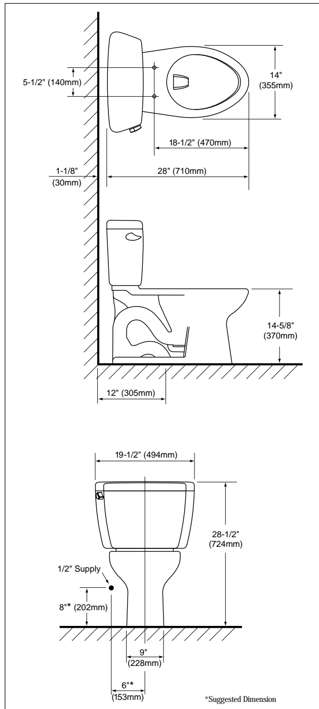
CST744EG - Eco Drake® Toilet
